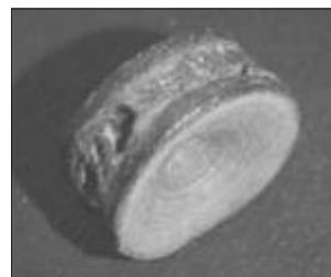
Vertèbre indéterminée - 22 mm
