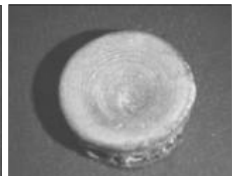
Vertèbre indéterminée - 22 mm
